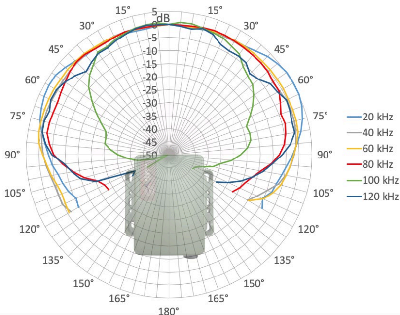
Song Meter Mini Bat Directionality (Vertical)
