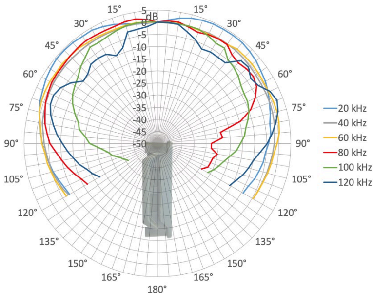
Song Meter Mini Bat Directionality (Vertical)
